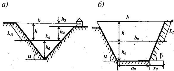
Рис. 4.1. Схема русла реки а – треугольное русло; б – трапецидальное русло
