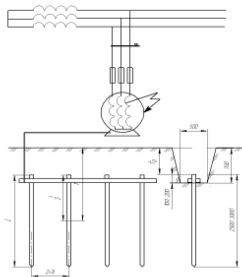
Рис. 3. Схема защитного заземления к примеру расчета
