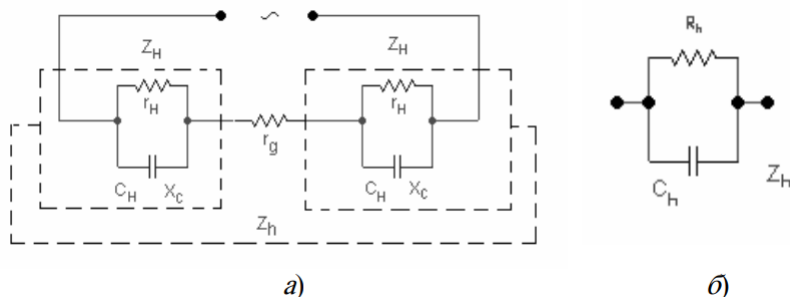
Рис. 15.1. Электрическая схема замещения тела человека (рука-рука): а – эквивалентная; б – упрощённая
