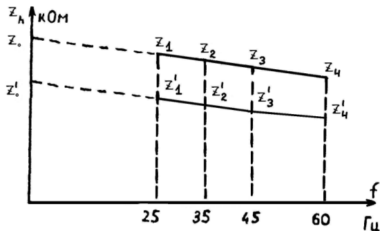
Рис. 15.2. График экстраполяции при определении сопротивления тела человека постоянному току
